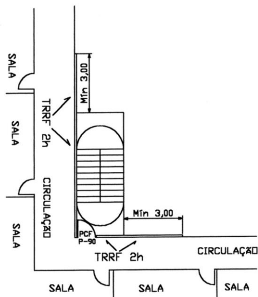
Figura 9 – Escada aberta externa
